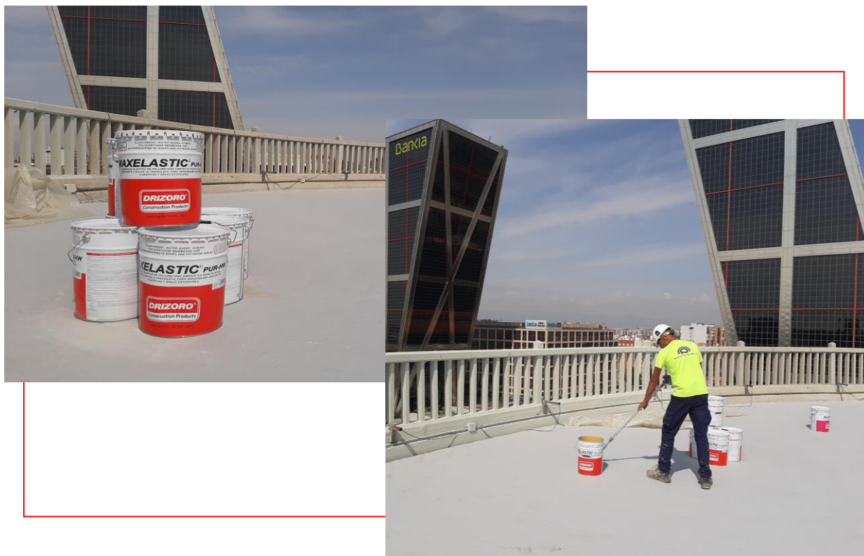
Impermeabilización de cubierta con el sistema MAXELASTIC® PUR -HW / Waterproofing of roof with MAXELASTIC® PUR -HW System
