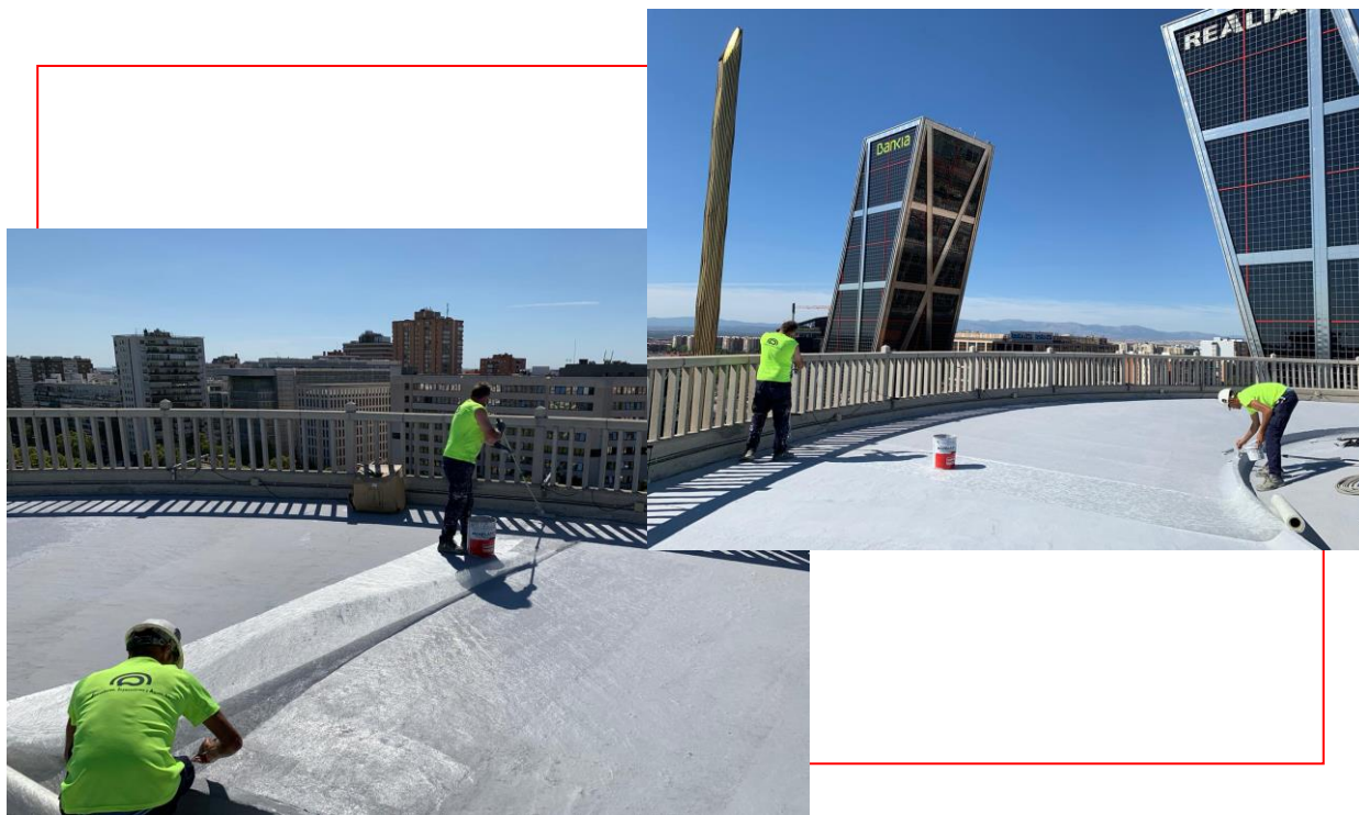
Aplicación de la primera capa de impermeabilización reforzada con velo de fibra de vidrio DRIZORO® VEIL M-100 / Application of first coat of the waterproofing system reinforced with glass fiber veil DRIZORO® VEIL M-100
